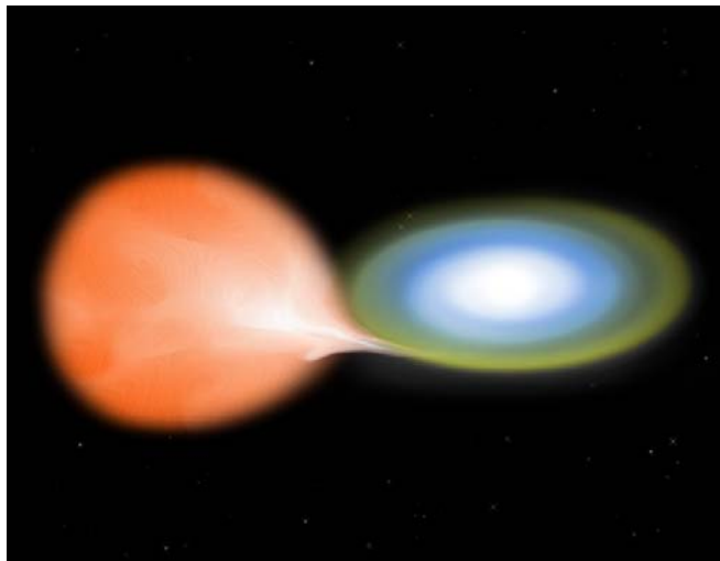
Kataklizmičke dvojne zvijezde u kojima je jedna od komponenata bijeli patuljak, neutronska zvijezda ili crna rupa vrlo su jaki izvori rendgenskog zračenja (vidi Okvir 2).
